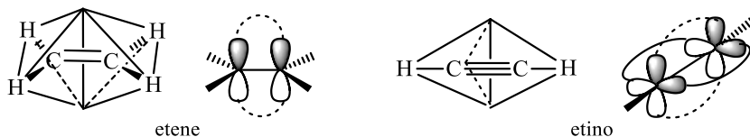
Figura 1.1. Costruzione dell'etene e dell'etino con carboni ibridati sp^3 .
