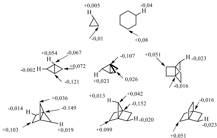
Figura 1.2. Distribuzione di carica su atomi di carbonio e di idrogeno di alcuni sistemi ciclici tensionati.
